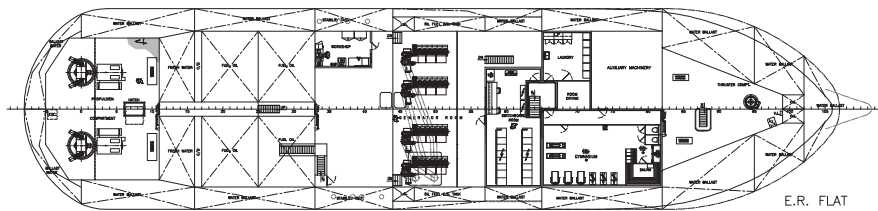
E.R. FLAT
